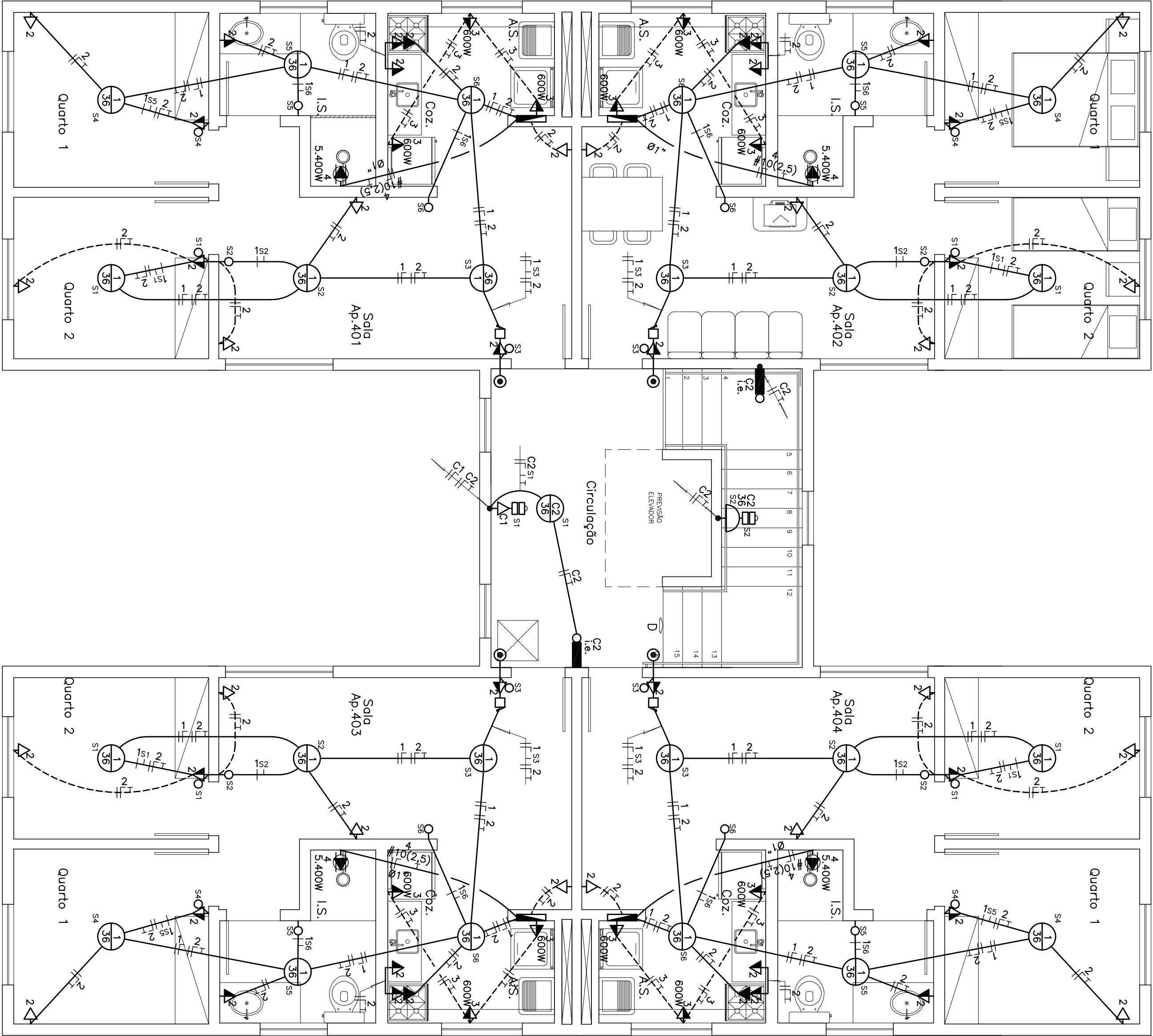
PLANTA 4º PAVIMENTO ESCALA 1 : 50
